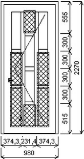
Vchodové dveře
